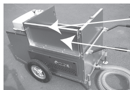
投雪パネル 前側への 取り付け
